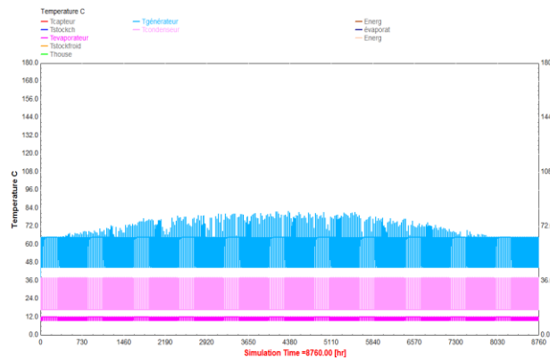
FIGURE 5. Températures des différents organes de la machine
