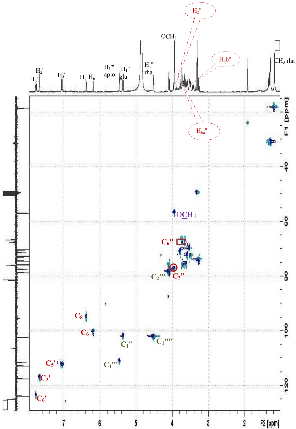
شكل 6: طيف تجارب HMQC للمركب A_2
