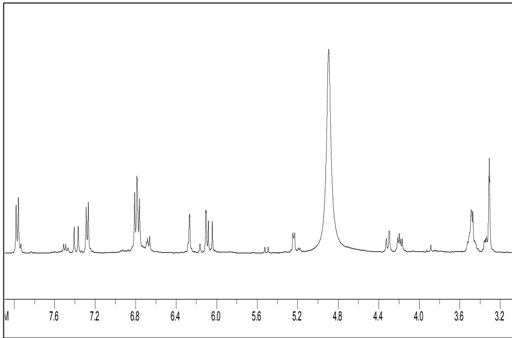
شكل 2: طيف ^1\text{H} RMN للمركب 4e
