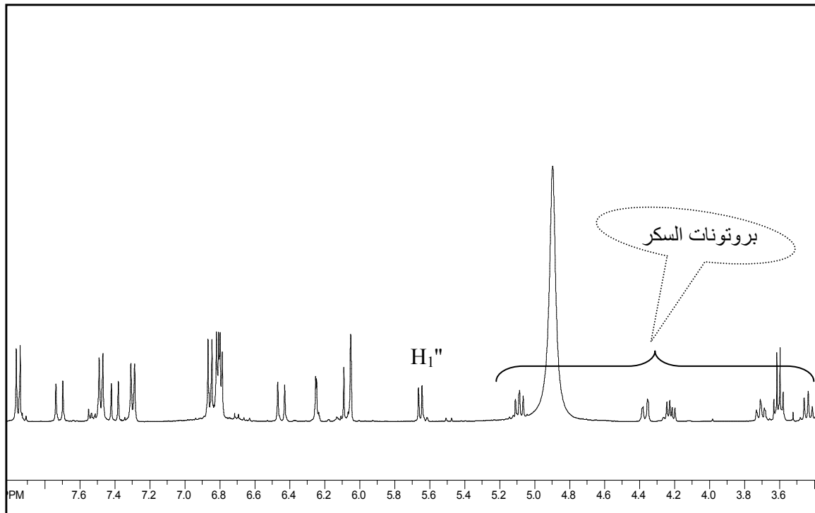
شكل 2: طيف ^1\text{H} RMN للمركب 5e
