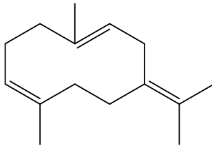
Germacrène B
