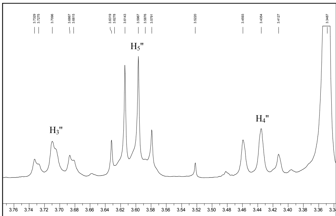
شكل 7 : طيف ^1\text{H} RMN للمركب
