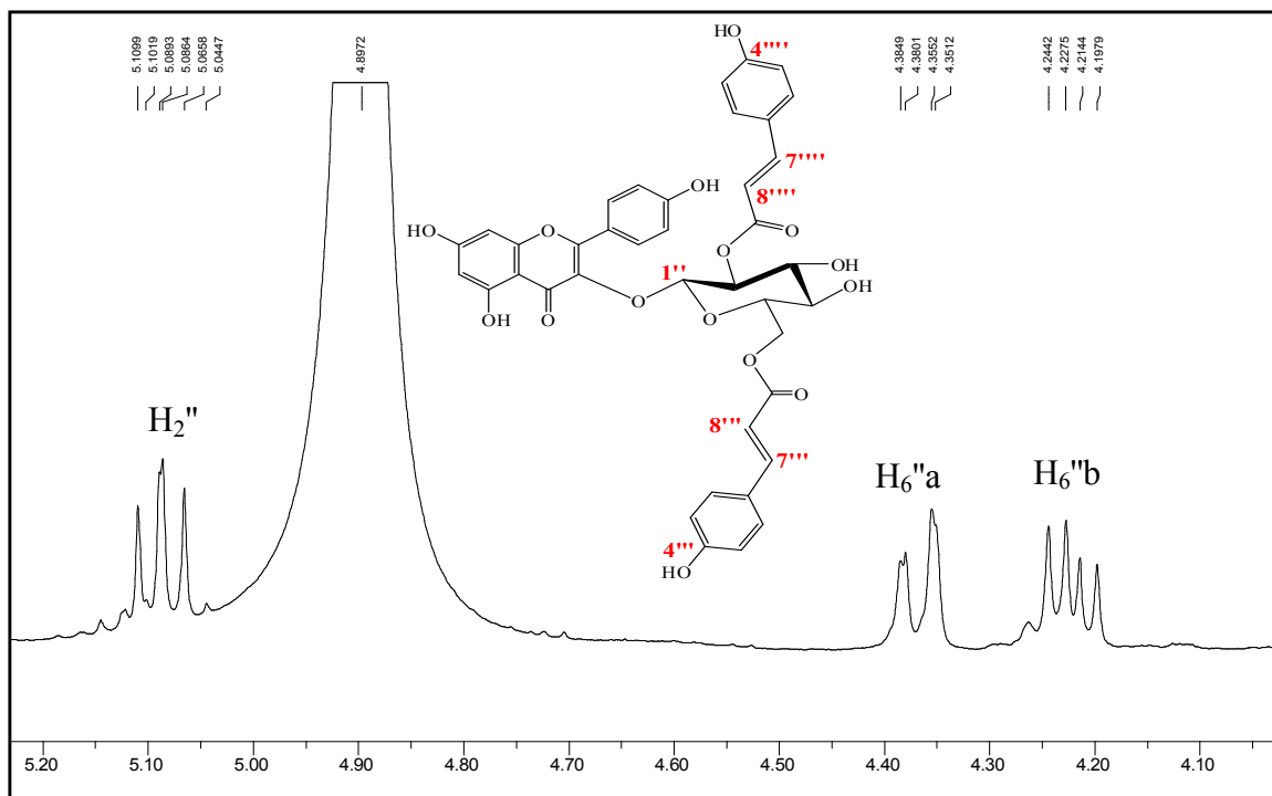
شكل 6 : طيف ^1\text{H} RMN للمركب
